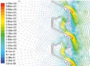
Uitblaas
